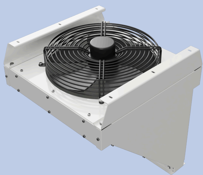
CA650 Largura: 650mm Peso: 30Kg Tensão: 220V/380V trifásico Velocidade do ar: 21m/s
